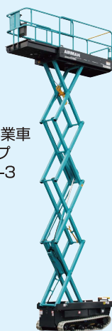
自走式高所作業車 クローラタイプ SR-128
